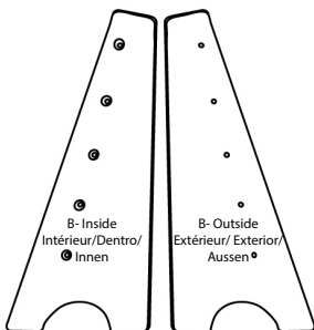
B - Left Panel (1x) Panneau Gauche / Panel Izquierdo / Linke Seite
