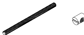
4 X WB 6/100 Gewindebolzen Threaded bolt Goujon fileté Clavija Barre filettate Tapbout
